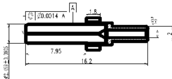
Figure-4:Ferrule
